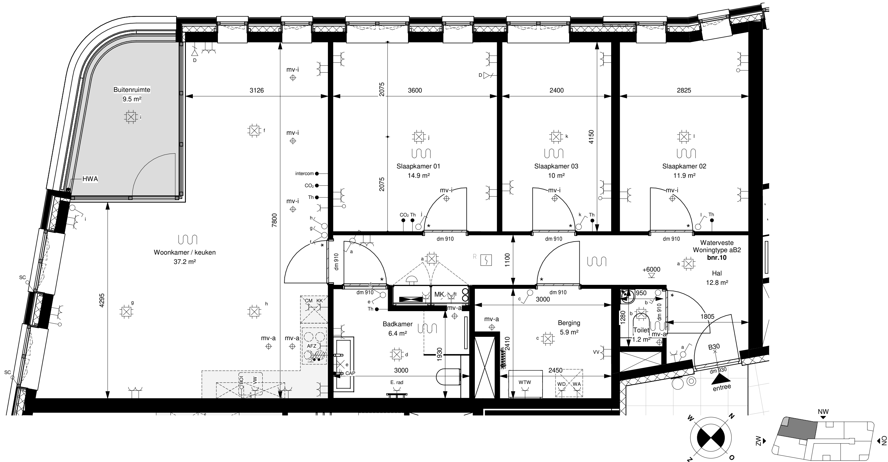
Plattegrond Schaal 1 : 50
